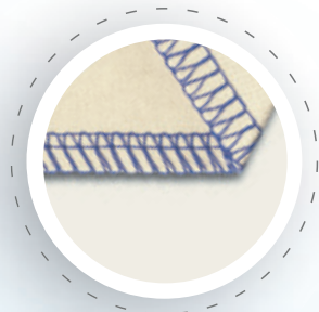
Point de surjet 4 fils Couture solide pour l'assemblage de la plupart des tissus
